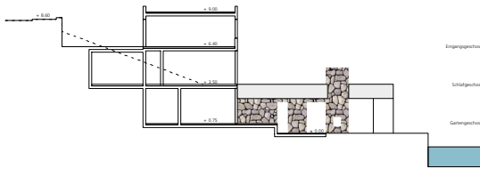
Querschnitt 1:500
