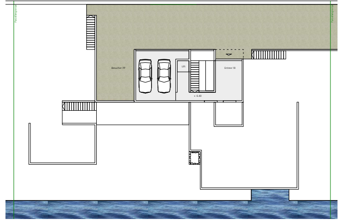
Grundriss Eingangsgeschoss 1:500
