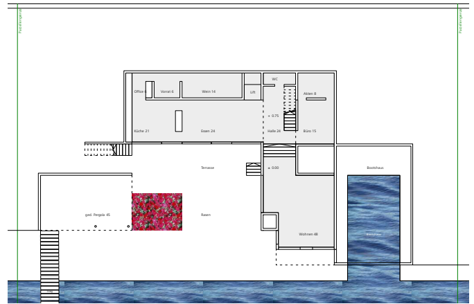
Grundriss Gartengeschoss 1:500
